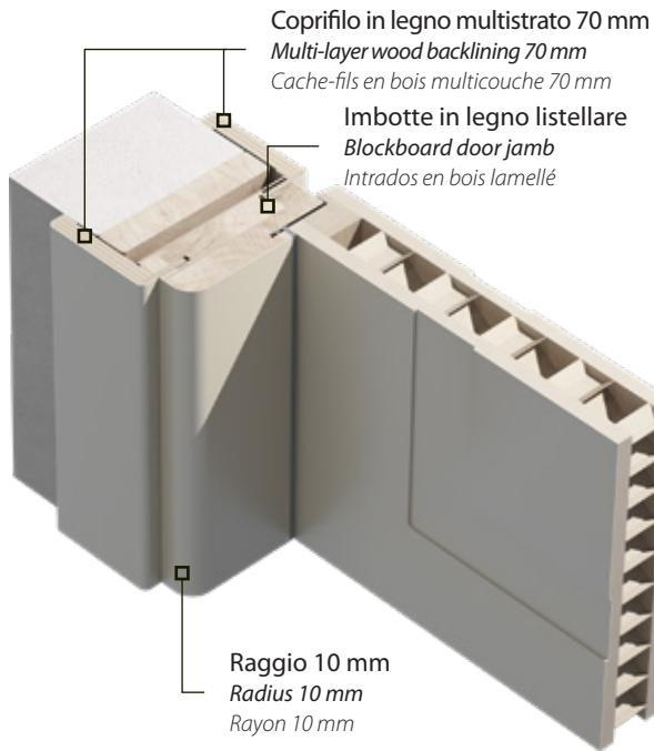
Imbotte - Raggio 10 con cerniera anuba (Standard)* Door jamb - Radius 10 with anuba hinge (Standard)* Intrados - Rayon 10 avec charnière anuba (Standard)*
