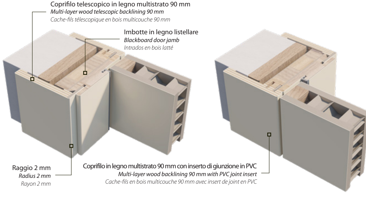
Imbotte - Raggio 2 con cerniera a bilico Door jamb - Radius 2 door jamb with pivot hinge Intrados - Rayon 2 avec charnière à pivot
