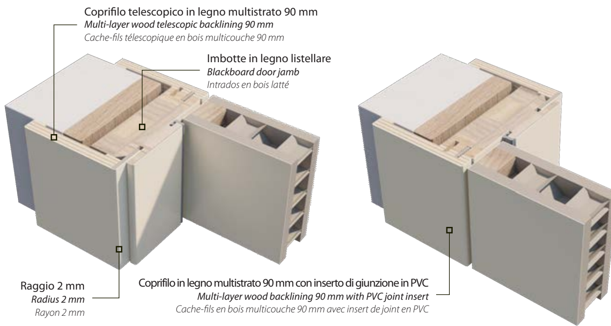
Imbotte - Raggio 2 con cerniera a scomparsa 3D MINIMAL Door jamb - Radius 2 with 3D hidden hinge MINIMAL Intrados - Rayon 2 avec charnière rétractable 3D MINIMAL
