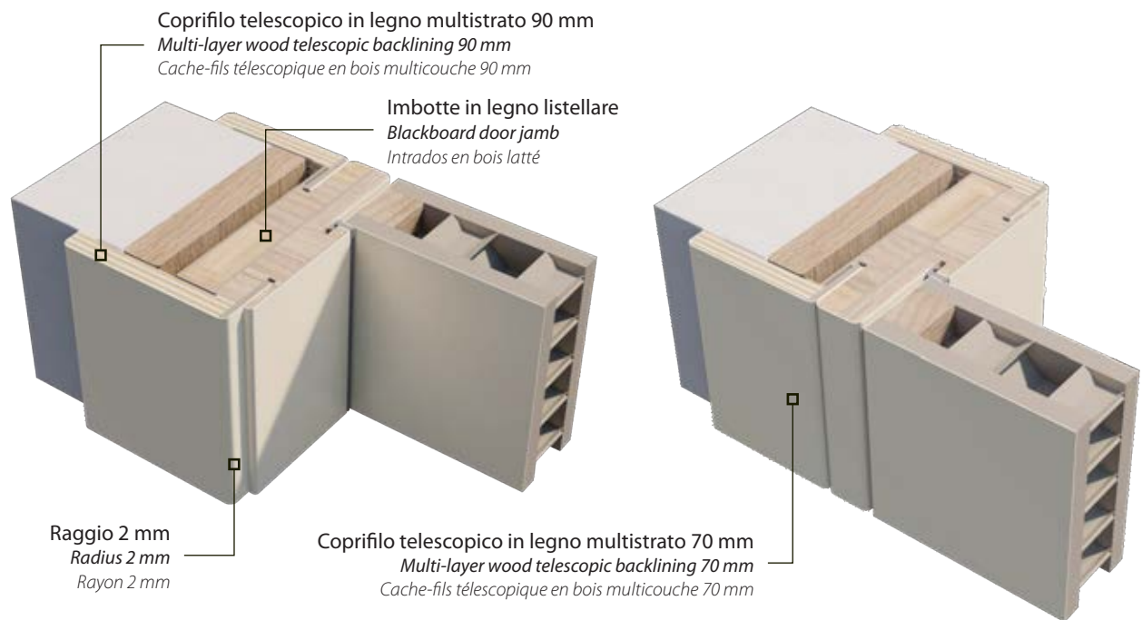
Imbotte - Raggio 2 con cerniera a scomparsa 3D MINIMAL Door jamb - Radius 2 with 3D hidden hinge MINIMAL Intrados - Rayon 2 avec charnière rétractable 3D MINIMAL
