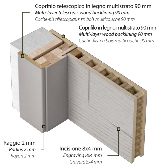
Imbotte - Raggio 2 con cerniera a scomparsa 3D MINIMAL Door jamb - Radius 2 with 3D hidden hinge MINIMAL Intrados - Rayon 2 avec charnière rétractable 3D MINIMAL
