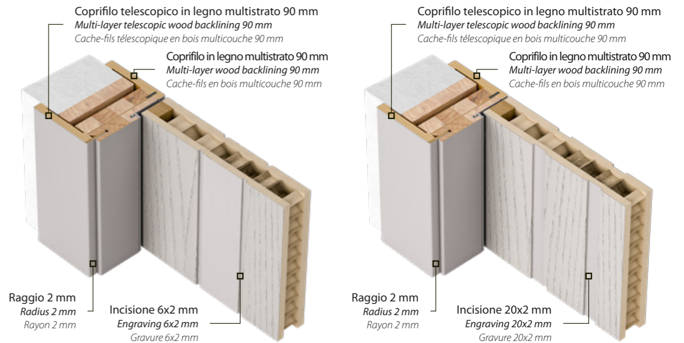
Imbotte Raggo 2 con cerniera a bilico Blackboard door jamb with pivot hinge Intrados en bois latté avec charnière à pivot
